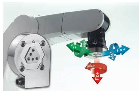
★ 新東工業の6軸力覚センサZYXer
